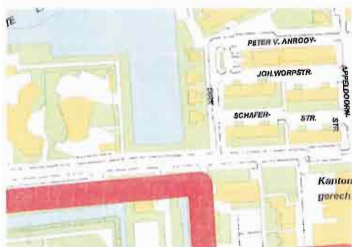
Figuur 25: Waterkering Fred Roeskøstraat.
